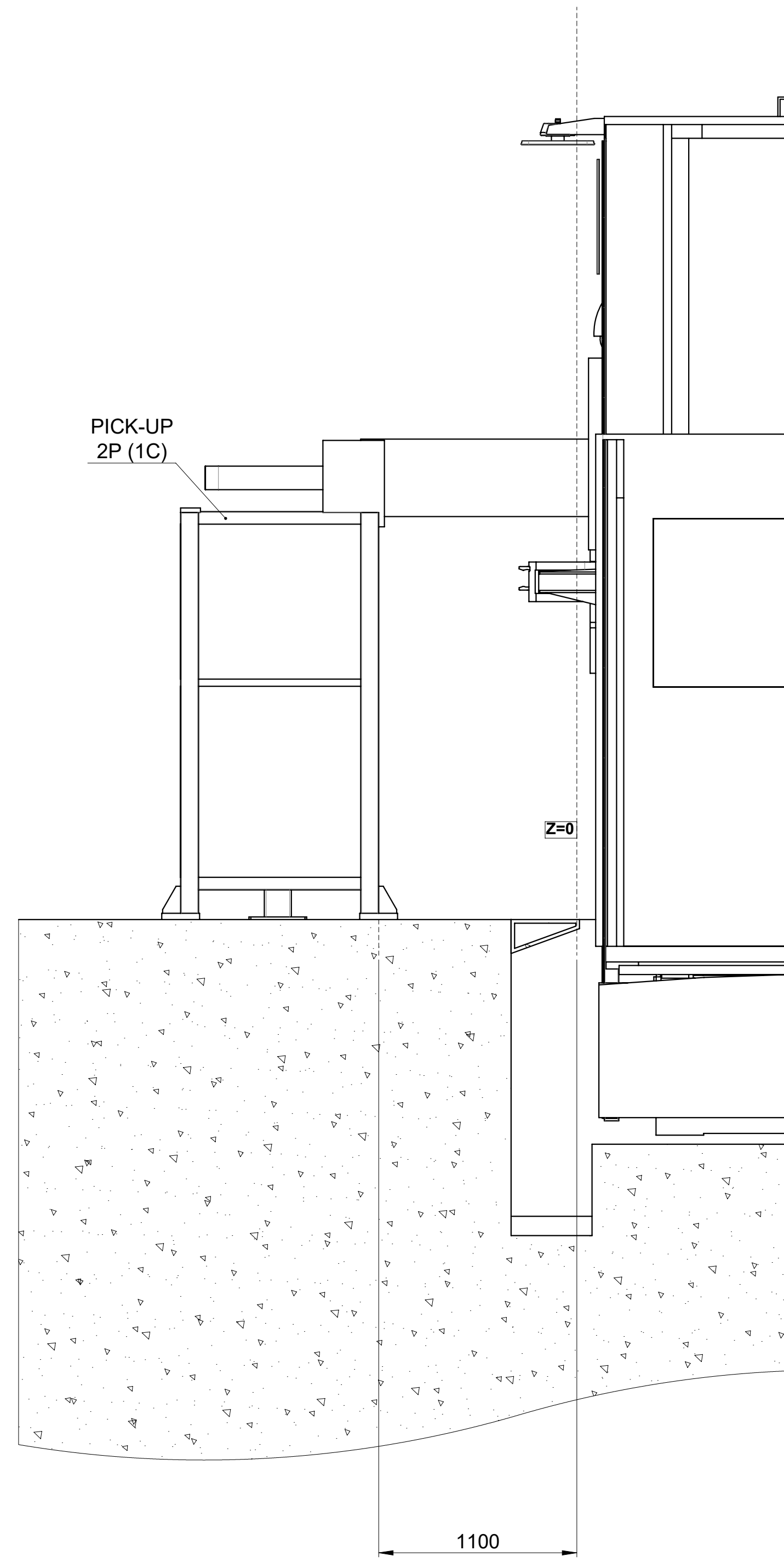
A-A 270°
