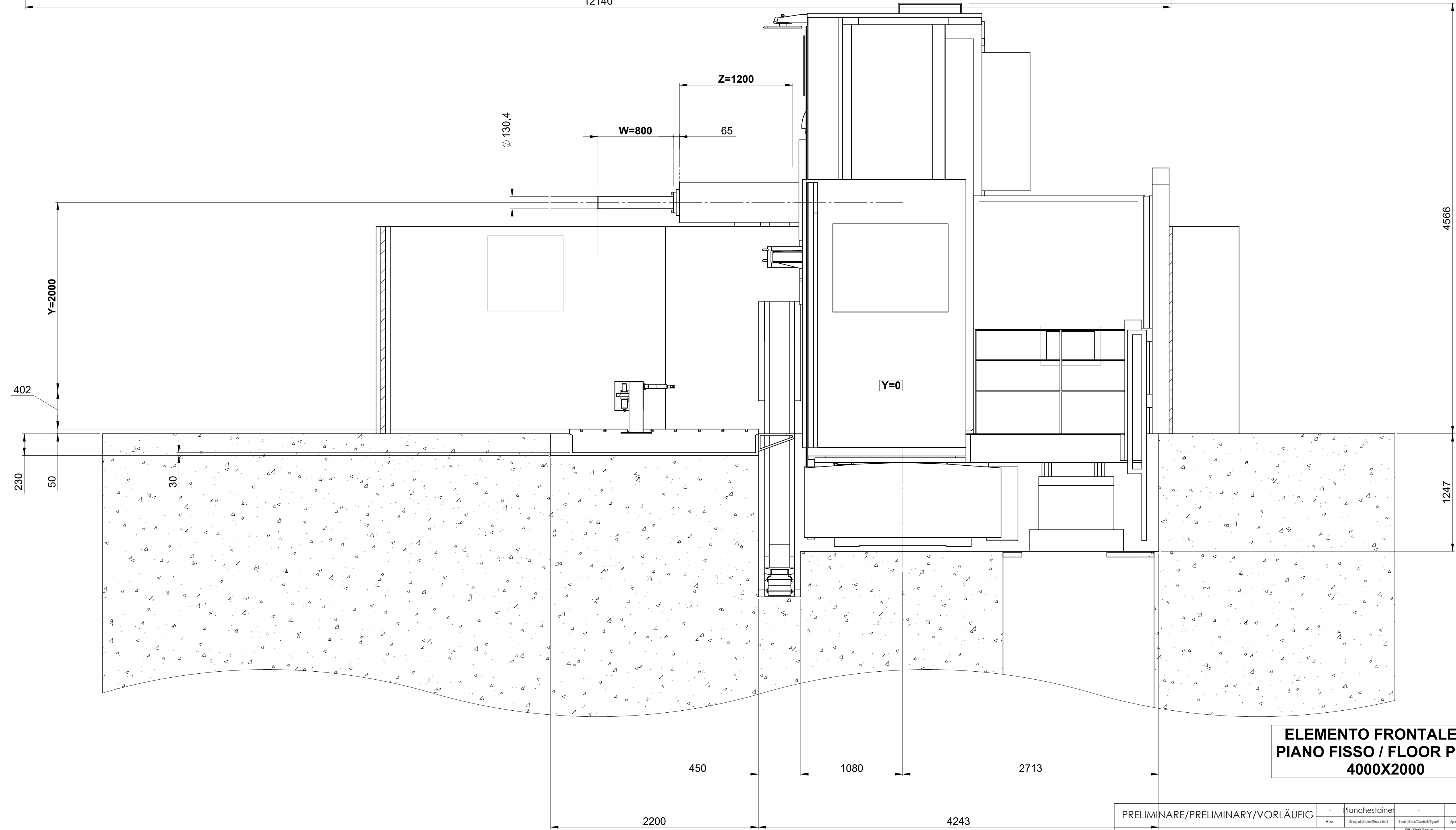
B-B 270°
